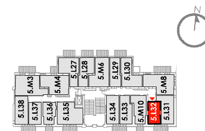
SCHEMAT KONDYGNACJI
